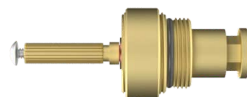
085118 REGISTRO ACQUASYSTEM, AMANCO X DECA DREAM Conversor para Registro AcquaSystem X Deca Dream, Polo e Level Antigo e Atual Estria: Deca Dream Rosca: N° 37 Sede: 36mm PPR: 20mm
