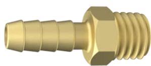
170502 | Saída Externa: TM 1/4" 170503 | Saída Externa: TM 5/16" ESPIGÃO NPT X TM Rosca Externa: NPT 1/4" Acabamento: Amarelo Material: Latão
