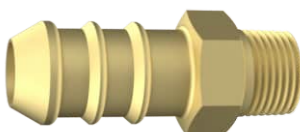
170500 Amarelo ESPIGÃO NPT X TM Saída Externa: TM 3/8" Rosca Externa: NPT 1/8" Material: Latão
