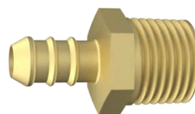
170501 | Saída Externa: TM 3/8" 170504 | Saída Externa: TM 5/16" 170505 | Saída Externa: TM 1/2" ESPIGÃO NPT X TM Rosca Externa: NPT 1/2" Acabamento: Amarelo Material: Latão
